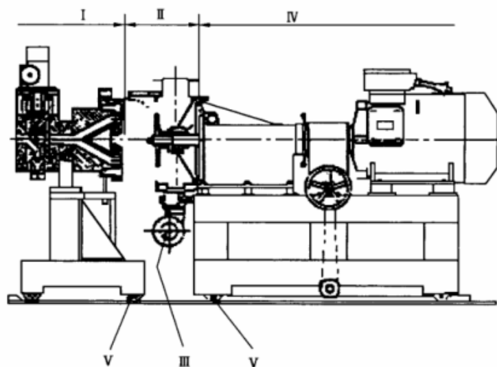
图 1 干法切粒机主要危险区示例
